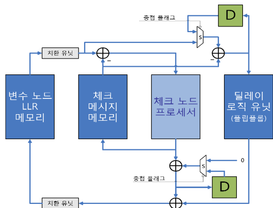
그림 12. 기본 구조와 중첩 구조를 동시에 지원하기 위하여 변경된 복호기 구조
