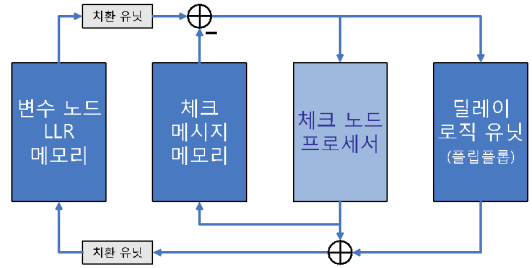
그림 7. 병렬 처리를 지원하는 기존 복호기의 구조
