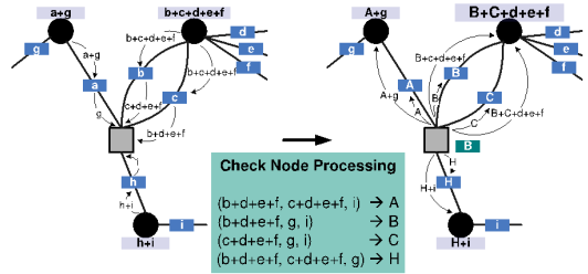
그림 11. 다중 중첩 구조를 지원하는 새로운 복호 방식
