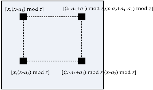
그림 3. 단일 블록 내에서 거스 4가 발생하는 경우 I
