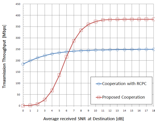
그림 7. 협력 통신 기법에 따른 transmission throughput (LOS와 NLOS가 함께 있는 경우)
