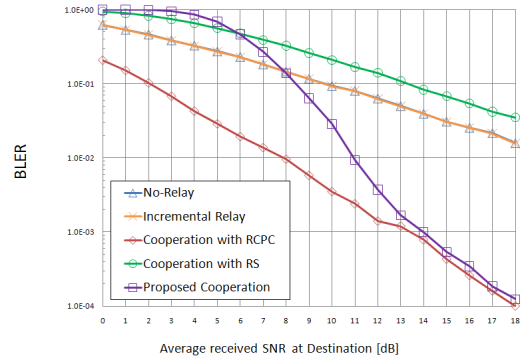
그림 4. 협력 통신 기법에 따른 BLER 비교 (LOS가 항상 존재하는 경우)
