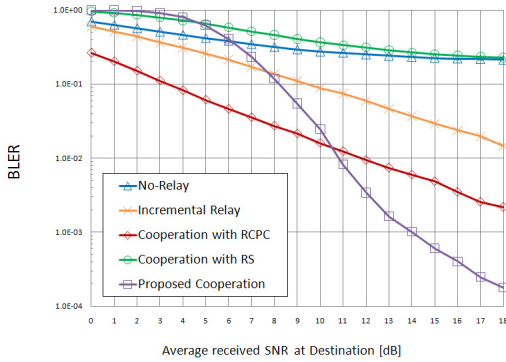
그림 6. 협력 통신 기법에 따른 BLER 비교 (LOS와 NLOS가 함께 있는 경우)
