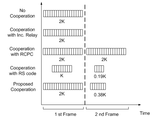
그림 3. 협력 통신 기법들의 데이터 전송 (LOS가 존재하는 환경)
