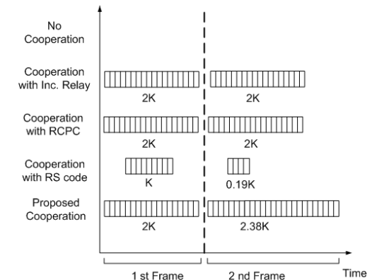
그림 4. 협력 통신 기법들의 데이터 전송 (LOS가 존재하지 않는 환경)
