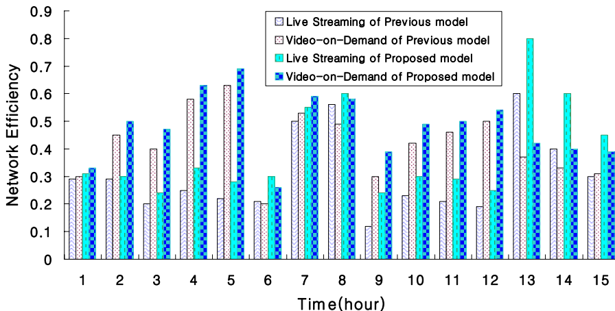
그림 5. 네트워크 효율성
