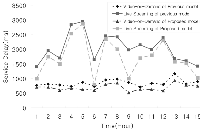
그림 7. 서비스 지연
