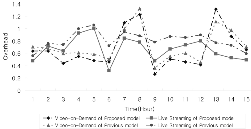
그림 6. 통신 오버헤드
