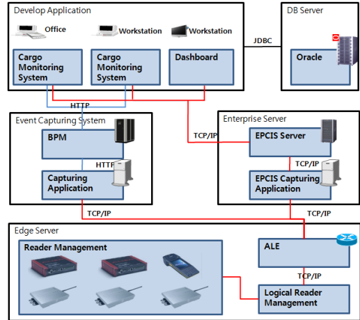
그림 1. AIDC 기술 기반 항공화물 모니터링 시스템 구성도
