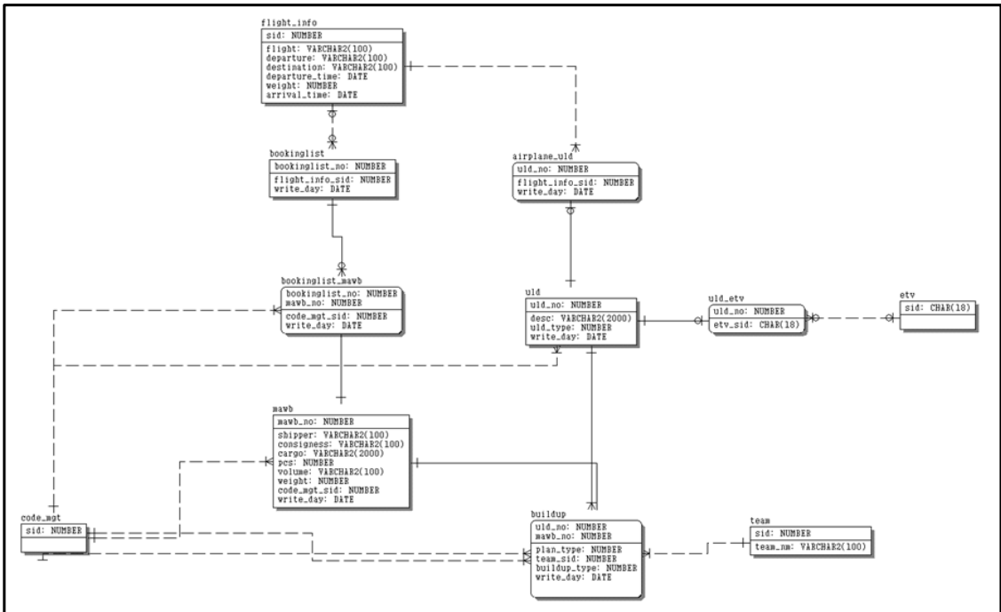
그림 3. 항공화물 모니터링 시스템의 Database 구조
