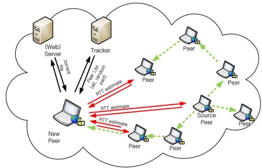
그림 1. 트래커 기반 P2P IPTV 구조
