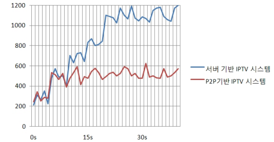
그림 16. 서버 기반 IPTV와 P2P 기반 IPTV 패킷량
