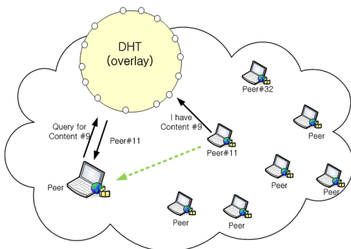
그림 3. DHT기반 P2P IPTV 구조
