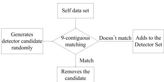
그림 8. 검출기 집합 생성 메커니즘 Fig. 8. Detector Set Generation
