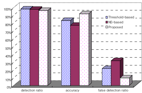
그림 16. 공격 탐지 기법들의 성능 비교 Fig. 16. Performance Comparison of Detection Schemes
