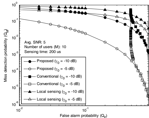
그림 2. \overline{\gamma} = -10, -5 dB일 때 제안 기법의 ROC Fig. 2. The complementary ROC curve of the proposed scheme when \overline{\gamma} = -10 and -5 dB
