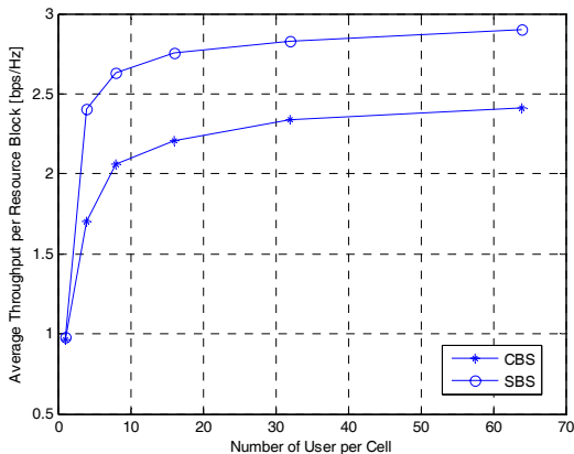
그림 4. 셀당 단말수에 따른 RB당 평균 데이터 전송율 Fig. 4. Average cell throughput per RB according to number of users per cell
