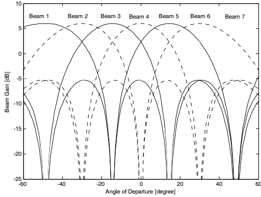
그림 2. 코드북에 사용된 프리코더들의 빔패턴 Fig. 2. Beam patterns of precoders in codebook
