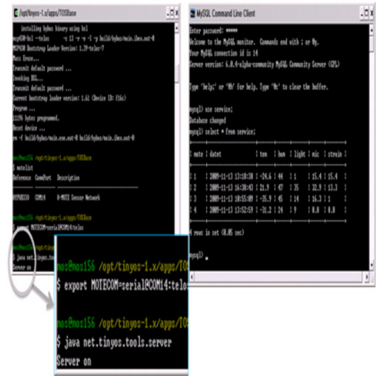
그림 6. 위치 센서 데이터의 데이터베이스 저장과정
