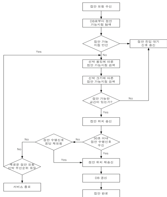
그림 4. 관제시스템의 접안유도과정 흐름도
