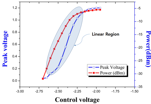
그림 10. Control Voltage에 따른 선형 구간 (약 -2.3V ~ 2.6V Control Voltage)
