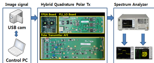
그림 11. 하이브리드 직교 폴라 송신 플랫폼 성능 분석 구성도 (영상 신호 수신, 하이브리드 직교 폴라 변조, 성능 측정 및 분석)
