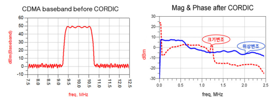
그림 2. 표준 CDMA 스펙트럼 (좌), CORDIC 알고리즘에 의해 분리된 크기 변조 신호와 위상 변조 신호 (우)
