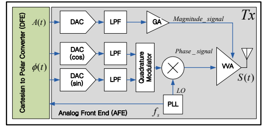
그림 8. 제안된 하이브리드 직교 폴라 송신 플랫폼 블록 다이어그램 (Digital Front End, Analog Front End)
