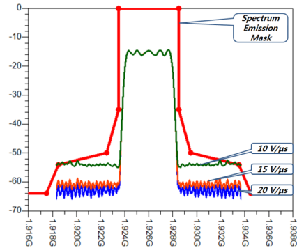
그림 5. 10, 15 그리고 20 V/μsec의 슬루율에 따른 WCDMA 스펙트럼 특성 (dBm/30 KHz RBW, 10 dB/div, 10 bit DAC, 1926 MHz 반송파)
