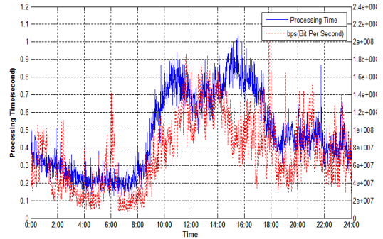
그림 9. 분류기 Processing Time 및 트래이스 bps Fig. 9. Identification system Processing Time, Trace bps
