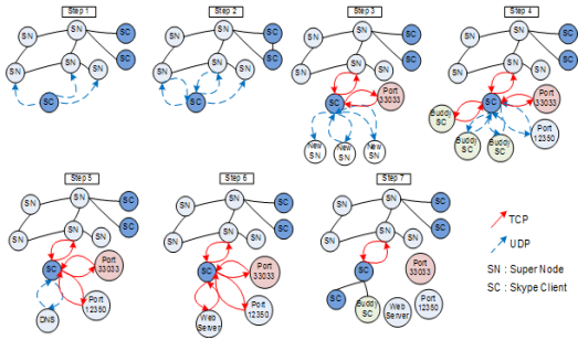
그림 2. Skype 응용의 Login 단계 Fig. 2. Skype Application Login Step
