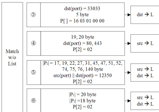
그림 5. 리스트를 사용하여 매칭 Fig. 5. Match w/o List
