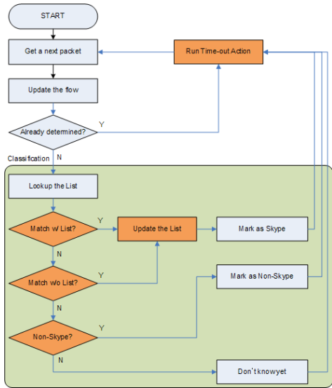
그림 3. 탐지 알고리즘 순서도 Fig. 3. Identification Algorithm Flow Chart
