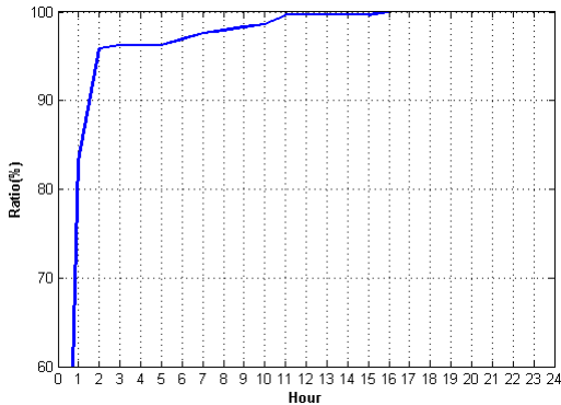
그림 7. Skype 호스트당 접속 유지시간 분포 Fig. 7. Distribution of Skype host connect time
