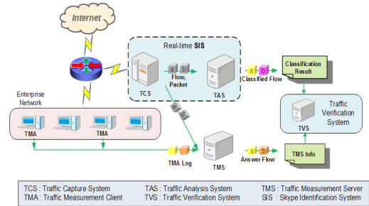
그림 1. 트래픽 수집 및 검증 시스템 Fig. 1. Traffic Collection, Verification System
