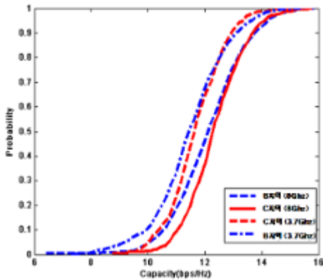
그림 7. 주파수별 전송 용량 비교 Fig 7. frequency transmission capacity comparison
