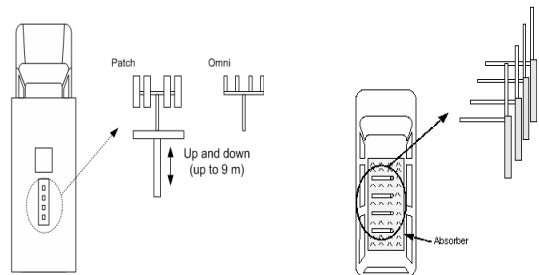
그림 2. MIMO 송수신 측정시스템의 개요도 Fig 2. MIMO transmission/reception measurement system block
