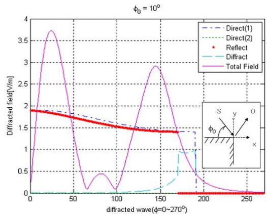
그림 6. 전계의 연속성 모의실험 결과 (0.5λ, φ 0 =10°, 20λ) Fig 6. electric field continuity simulation result(0.5λ, φ 0 =10°, 20λ)
