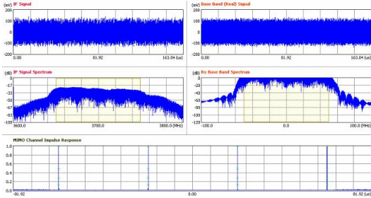
그림 10. 채널 사운드의 기저대역 및 계측기 검출신호 파형 Fig 10. Channel sound sink band and measurement signal wave
