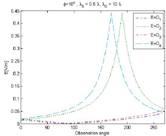
그림 5. 전계의 연속성 모의실험 결과 (0.5λ, φ 0 =10°, 10 λ) Fig 5. electric field continuity simulation result(0.5λ, φ 0 =10°, 10 λ)
