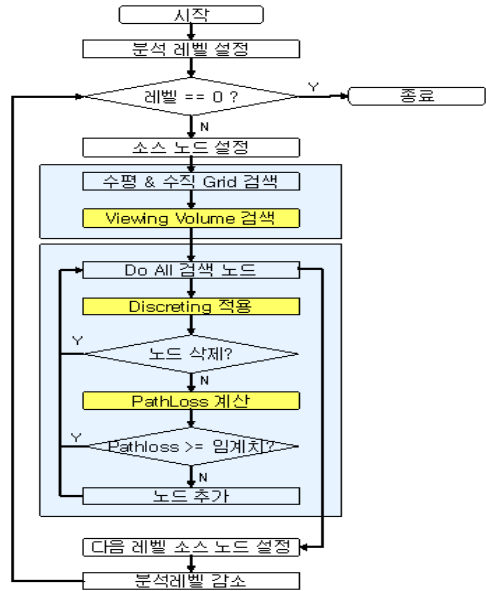
그림 3. 예측분석을 위한 트리생성 알고리즘 개념도 Fig 3. forecast analysis for terr generation algorithm block
