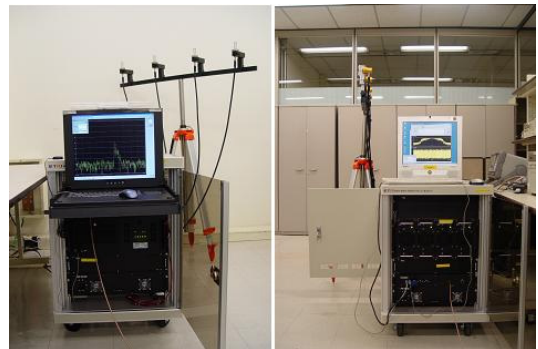
그림 1. MIMO 채널 사운드러 사진 Fig 1. MIMO Channel sounder photograph
