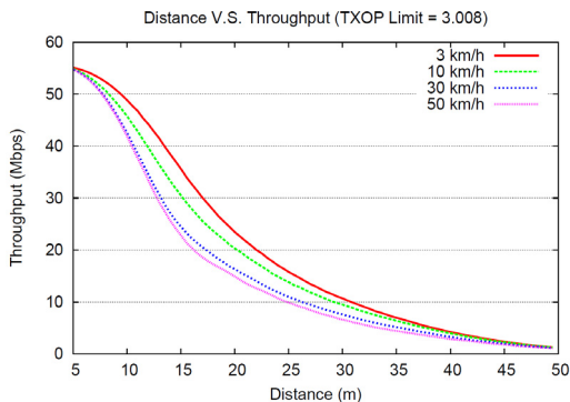
그림 2. Distance vs. throughput (TXOP Limit: 3.008 msec).
