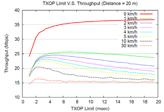
그림 3. TXOP Limit vs. throughput (Distance: 20 m).
