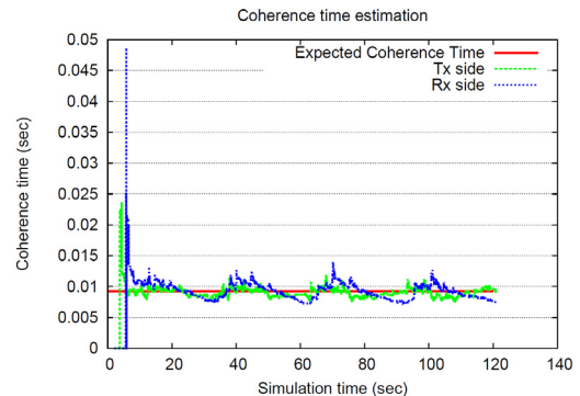
그림 9. 단말이 움직이는 환경에서의 coherence time 추정.
