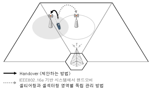
그림 8. IEEE802.16e 기반 시스템에서의 핸드오버와 제안하는 셀 관리 방법에서의 핸드오버 비교
