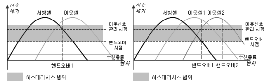
그림 4. IEEE802.16e시스템에서 중첩된 셀의 핸드오버
