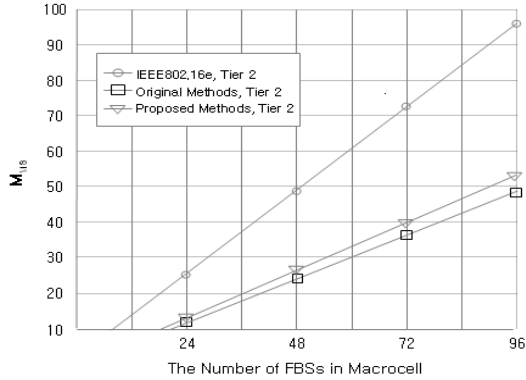
그림 12. 매크로셀 구역(섹터링)과 셀 내 FBS수에 따른 MMS의 변화
