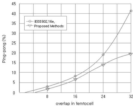
그림 14. 단말기에 중첩된 펠토셀이 증가함에 따른 핑퐁 발생률
