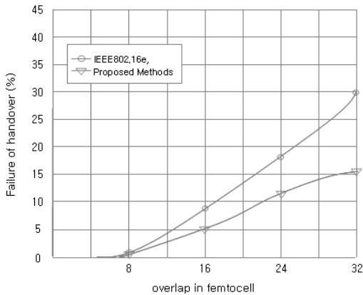
그림 15. 단말기에 중첩된 펠토셀이 증가함에 따른 핸드오버 실패율
