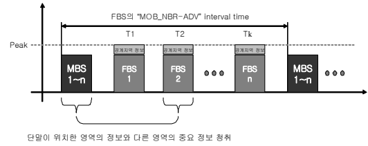
그림 7. 제안된 MOB_NBR-ADV (단말은 자신이 위치한 영역과 경계지역의 정보 획득)
