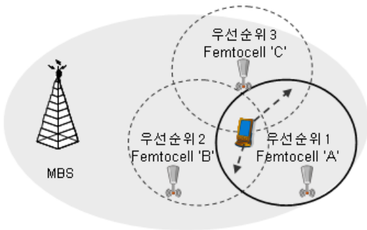
그림 11. 제안된 우선순위 셀별 차등적 핸드오버
