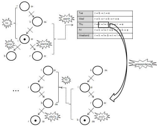
그림 6. 에러 발생시 연속적인 매칭 알고리즘 수행방식
