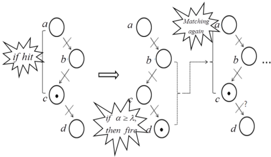
그림 4. 시간 페트리 넷을 사용한 연속적인 매칭 알고리즘
