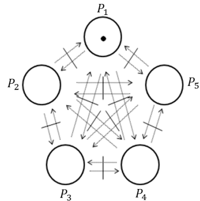
그림 3. 시간 페트리 넷이 적용된 장소
