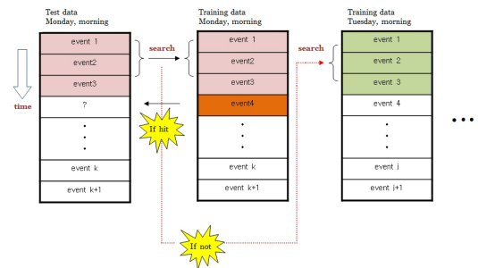
그림 1. 지능형 순차적 매칭 알고리즘의 개념도
