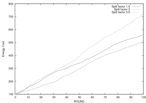
그림 15. Split factor를 달리하였을 때의 에너지 소모량
