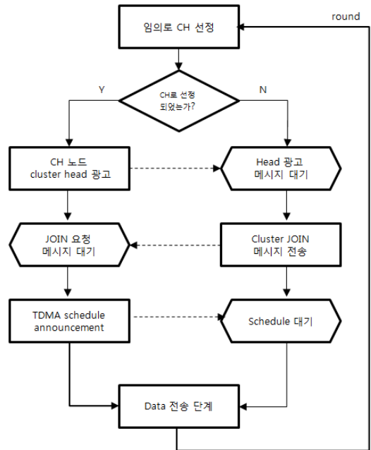
그림 1. LEACH 순서도
