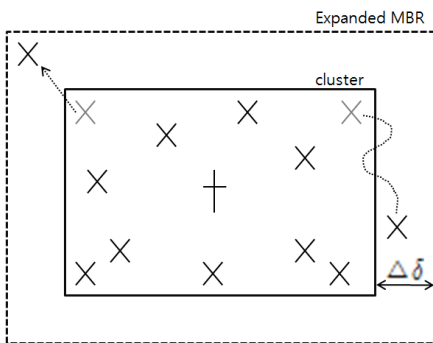
그림 7. Expanded MBR
