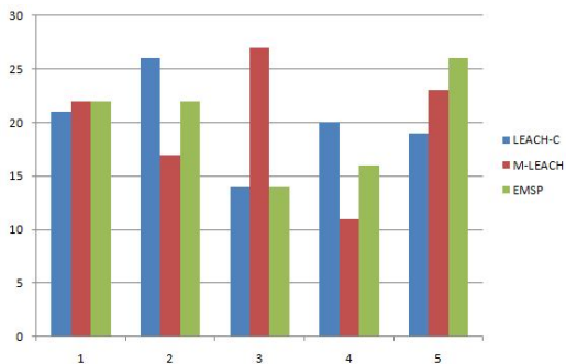
그림 12. Invitation phase 후의 각각의 클러스터 내의 노드의 수
