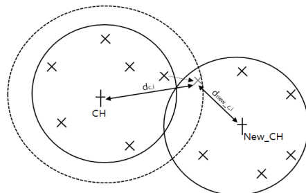
그림 8. virtual cluster
