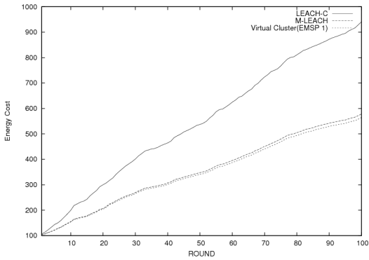
그림 10. 100개 노드에서의 100 round 동안의 에너지 소모량 비교
