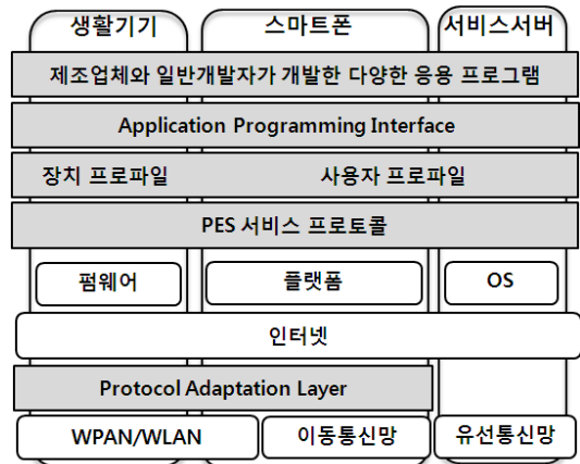
그림 4. PES 기본 프로토콜 구조
