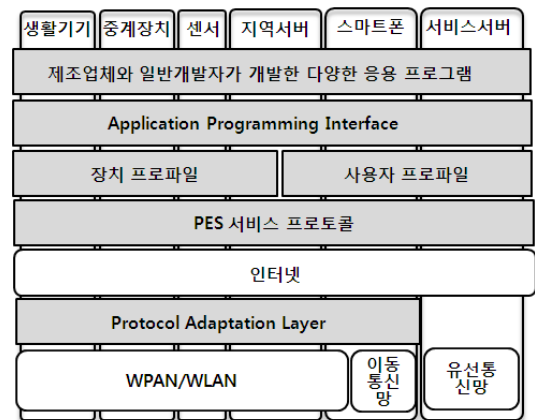
그림 6. 확장된 PES 프로토콜 구조
