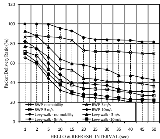
그림 6. 이동성 모델에 따른 OLSR 패킷 전달률 비교
