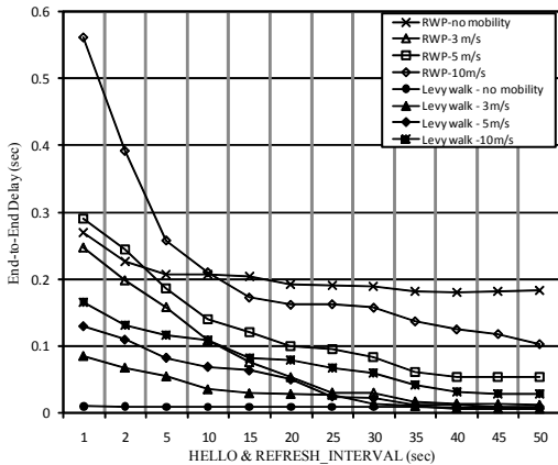
그림 8. 이동성 모델에 따른 OLSR 종단간 지연시간
