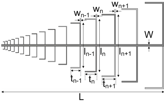
그림. 2 역-L 형태의 다이폴 소자로 구성된 LPDA 안테나 구조 Fig. 2. Geometry of an LPDA antenna with inverted-L shaped dipole elements.
