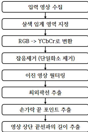
그림 2. 손가락 길이 추출 프로그램 흐름도
