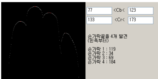
그림 14. 손끝 추출 및 길이 비교 결과 추출 영상
