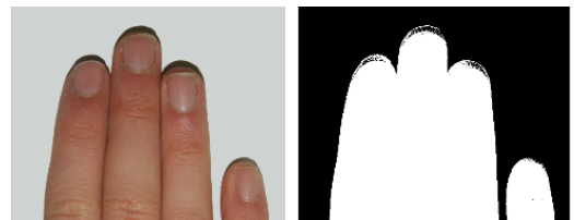
그림 6. 입력 영상
