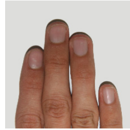
그림 15. 입력 영상
