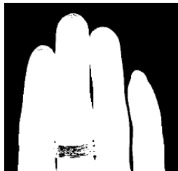
그림 13. 이진화 영상
