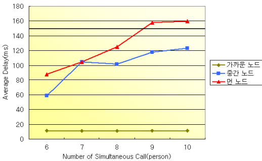
그림 6. 동시 통화자 수 변화에 따른 지연 변화 그래프
