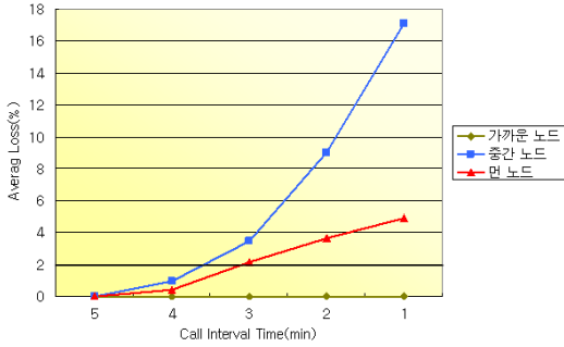
그림 5. CIT 변화에 따른 손실률 변화 그래프
