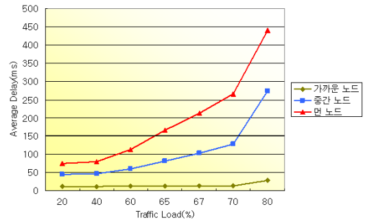
그림 8. Traffic load 변화에 따른 지연 변화 그래프
