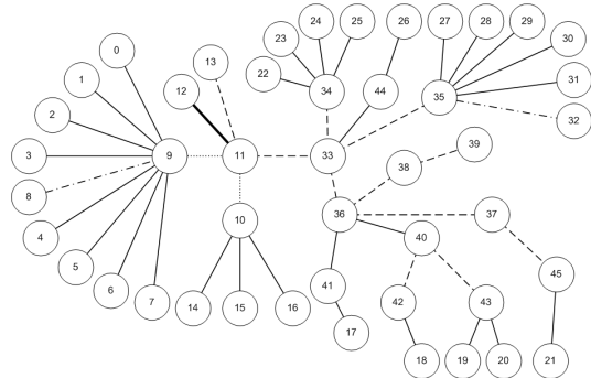
그림 1. 시뮬레이션 네트워크
