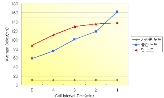
그림 4. CIT 변화에 따른 지연 변화 그래프
