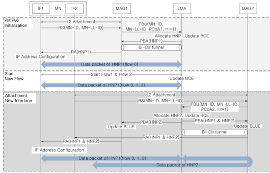
그림 1. 제한한 PMIPv6 시그널링 절차
