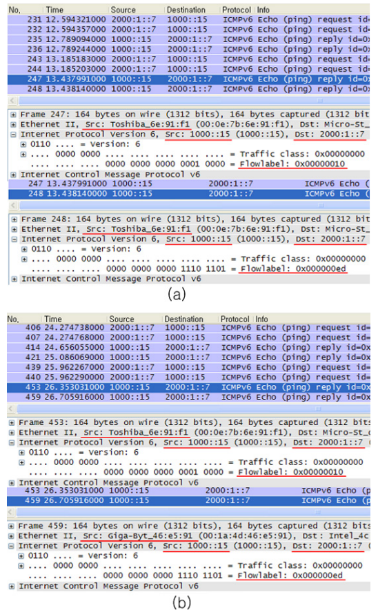
그림 4. MN 패킷 캡처 결과 (a) 플로우 핸드오버 전 (b) 플로우 핸드오버 후
