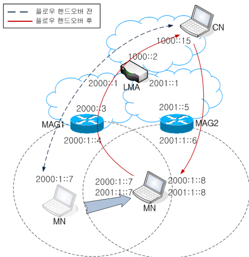
그림 3. 시험망 구성
