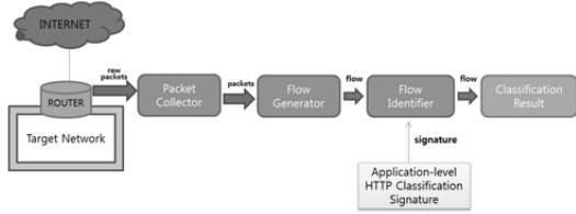
그림 1. HTTP 트래픽 분류 시스템 구조
