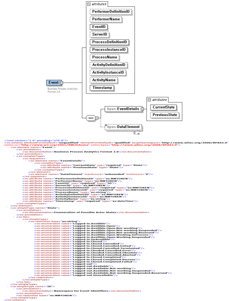
그림 6. 프로세스 모델의 업무수행자 실행이력이벤트로그포맷의 XML스키마 구조와 상세포맷
