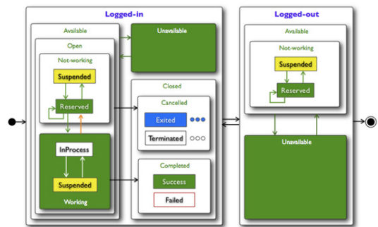
그림 5. 프로세스 모델의 업무수행자 실행시점 상태관리 모델
