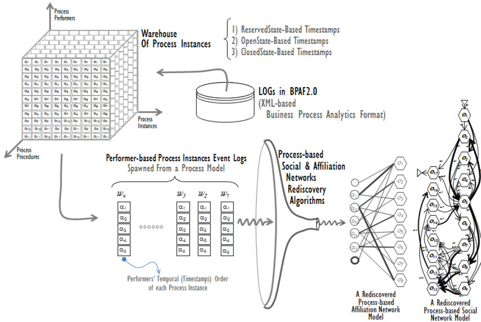
그림 7. BPAF2.0의 수행자 실행이력 이벤트로그표준포맷 기반의 소셜네트워크 및 소속성네트워크 재발견 프레임워크
