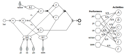
그림 3. 정보제어넷과 그의 실행이력 이벤트로그로부터 재발견(마이닝)한 소속성네트워크 예
