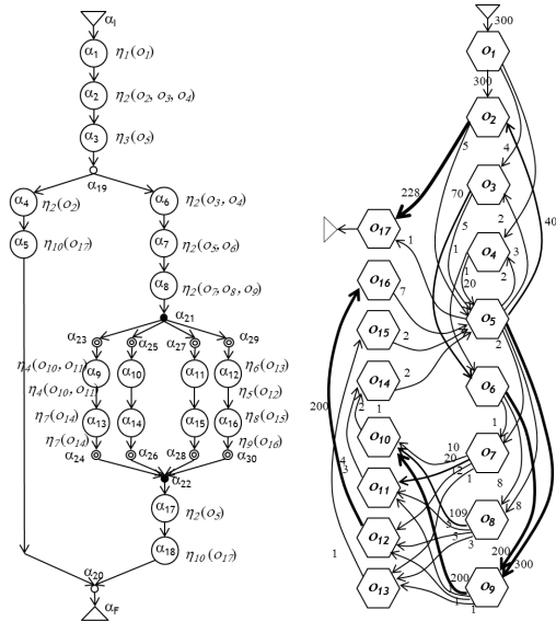
그림 2. 정보제어넷기반 프로세스 모델과 그의 실행이력 이벤트로그로부터 재발견(마이닝)한 소셜네트워크 예
