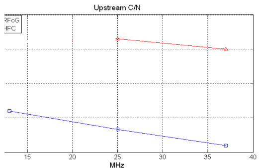
(b) RFoG / HFC 네트워크 상향 CNR
