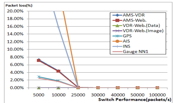
그림 6. 스위치 성능 별 패킷 손실률 Fig. 6. End-to-end packet loss ratio with respect to switching performance of integrated gateway
