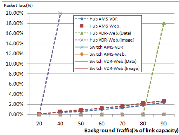
그림 4. 통합 게이트웨이의 망요소적 역할 및 백그라운드 트래픽 별 패킷 손실률 Fig. 4. Packet loss ratio with respect to background traffic and role of integrated gateway
