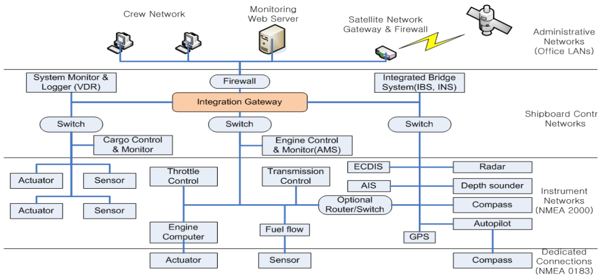
그림 2. 선박 통합 네트워크의 참조망 구조 Fig. 2. Reference network architecture of integrated ship area network
