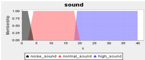
그림 5. 전진부 퍼지 소속도 함수 Fig. 5. Fuzzy membership function of antecedent.
