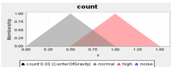
그림 6. 후진부 퍼지 소속도 함수 Fig. 6. Fuzzy membership function of consequent.
