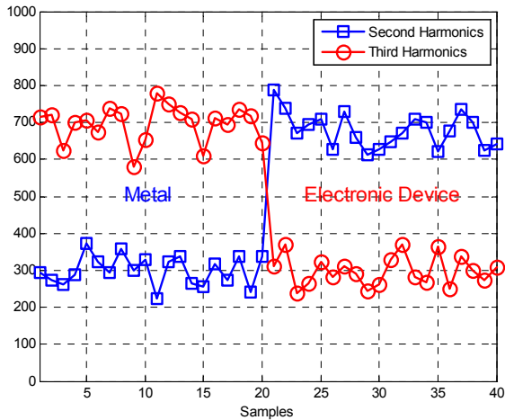
그림 2. 전자소자 탐지기의 ADC로부터 측정된 2차 및 3차 고조파 크기
