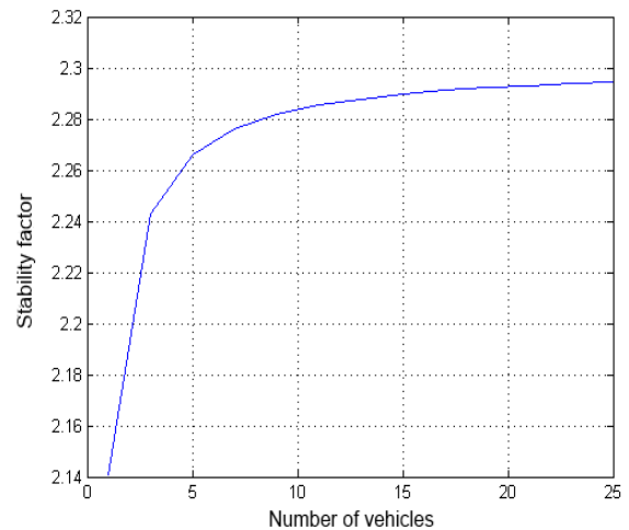
그림 5. 포화 상태에서의 안정성 지수 Fig. 5. Stability factor for the saturation case
