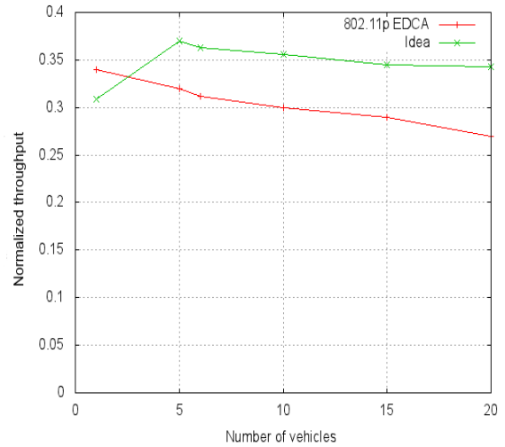
그림 4. 정규화 된 네트워크 처리량 비교 Fig. 4. Normalized networks throughput comparisons
