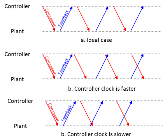
그림 2. 클럭동기화 문제점 Fig. 2. Problem of Clock Synchronization
