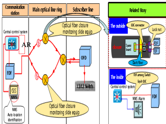
그림 1. 접속합체 감시 시스템 개황도 Fig. 1. Optical cable monitoring system functional block diagram
