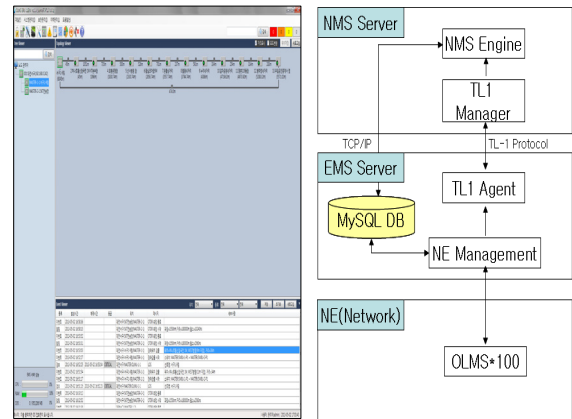
그림 7. 광케이블 접속함체 감시 NMS 화면 경보 내용 Fig. 7. Optical fiber closure monitoring NMS Screen contents of alarm [18]
