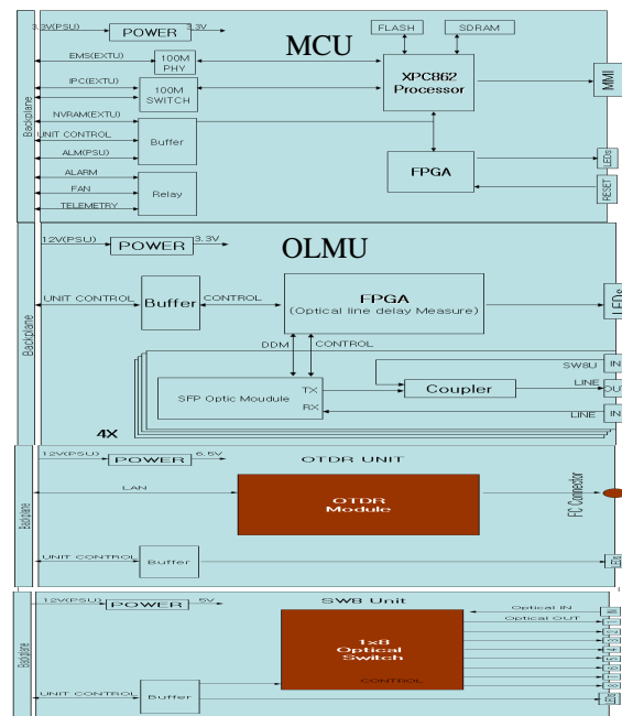
그림 8. 광선로 OLMS UNIT 구성도 Fig. 8. Optical Line Monitoring Unit block diagram [18]
