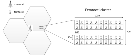
그림 2. 모의실험 환경 Fig. 2. Simulation model
