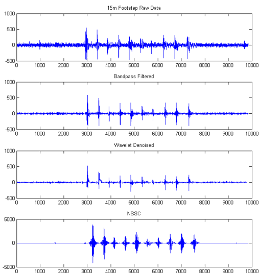
그림 14. 15미터, 맑은 날, 잡음 제거(Raw, BP, Wavelets, NSSC) Fig. 14. 15m, sunny day, noise subtraction (Raw, BP, Wavelets, NSSC)
