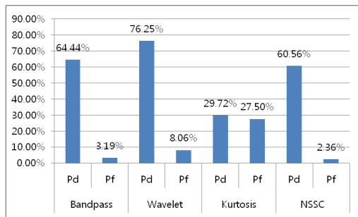
그림 17. 맑은 날(바람<0.5m/s) 탐지 및 오경보 확률 Fig. 17. Sunny day(wind<0.5m/s) Pd and Pf
