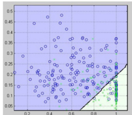
그림 12. LS방식을 이용한 식별 경계면 Fig. 12. Classification decision boundary using LS
