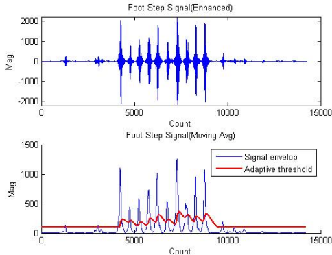
그림 8. NSS 처리 신호에 대한 적응 임계치 적용 Fig. 8. Adaptive threshold applying to NSSC processed signal
