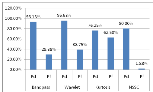
그림 18. 비오는 날(5mm/hour) 탐지 및 오경보 확률 Fig. 18. Rainy day(5mm/hour) Pd and Pf
