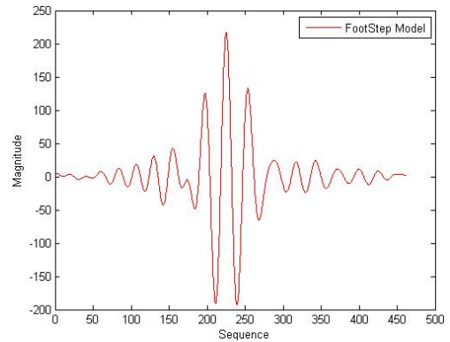
그림 6. 기본 발자국 모델 신호 파형 Fig. 6. Prime footstep model signal waveform
