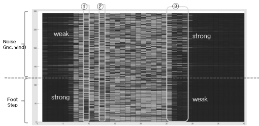
그림 10. 발자국과 잡음의 주파수 대역별 신호세기 Fig. 10. Power spectrum of footstep and noise
