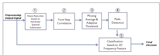
그림 2. 발자국 탐지과정 블록도 Fig. 2. Footstep detection procedure block diagram
