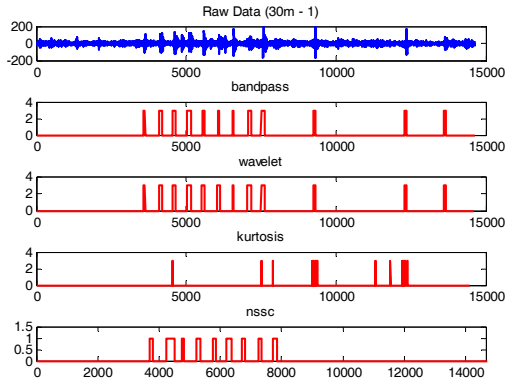
그림 16. 30미터, 비오는 날 탐지 결과(Raw, BP, Wavelets, Kurtosis, NSSC) Fig. 16. 30m, rainy day. detection result(Raw, BP, Wavelets, Kurtosis, NSSC)
