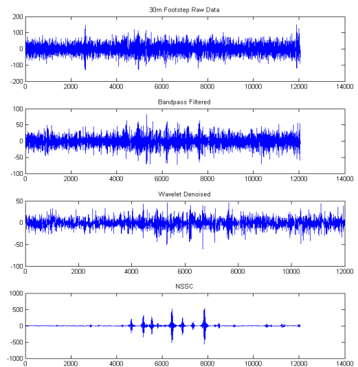
그림 15. 30미터, 맑은 날, 잡음 제거(Raw, BP, Wavelets, NSSC) Fig. 15. 30m, Sunny day, noise subtraction (Raw, BP, Wavelets, NSSC)
