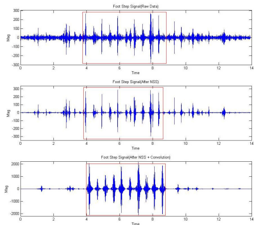
그림 7. 입력신호(맨위), NSS 처리후(중간), NSSC 처리후(맨아래) Fig. 7. Input Sig.(Top), After NSS (Mid), After NSSC (Bottom)
