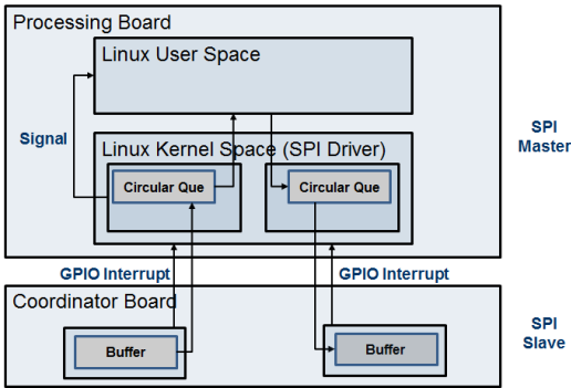
그림 6. 프로세싱 보드와 코디네이터 보드 연동을 위한 블록 다이어그램
