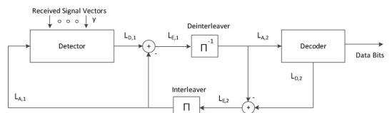
그림 3. 반복적인 검출 및 복호 수신기의 블록다이어그램 Fig. 3. A block diagram of iterative detecting and decoding receiver
