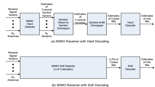
그림1. MIMO SM 수신기 Fig. 1. MIMO SM receiver
