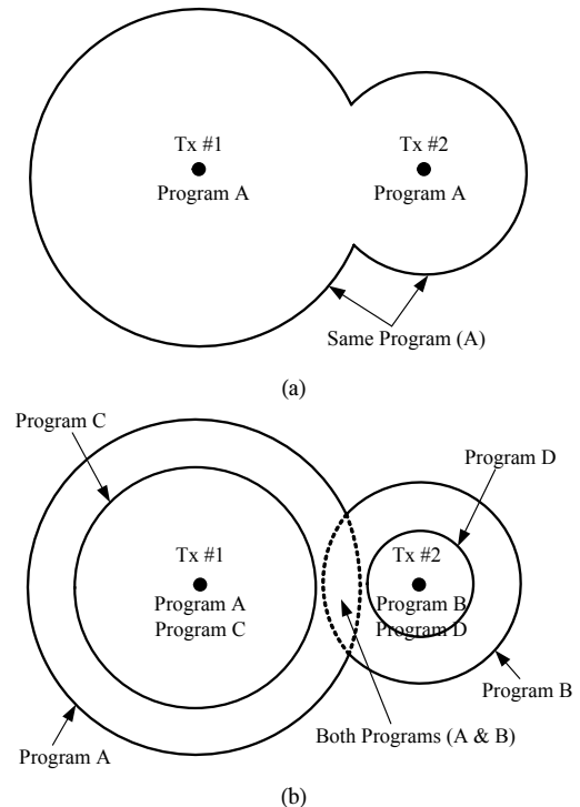
그림 1. 두 개의 방송 송신기에 대한 서비스 영역 7 . (a) 기존의 SFN. (b) 클라우드 전송 시스템 Fig. 1. Service coverages for two broadcasting transmitters 7 . (a) conventional SFN and (b) cloud transmission system
