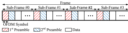
그림 2. 클라우드 방송 시스템을 위한 프레임 구조의 예 [11] Fig. 2. An example of the frame structure for cloud transmission systems [11] .
