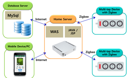
그림 1. 스마트 멀티탭 시스템의 전체 통신 개요도 Fig. 1. Overview of the entire communication system, a Smart Multiple-Tap
