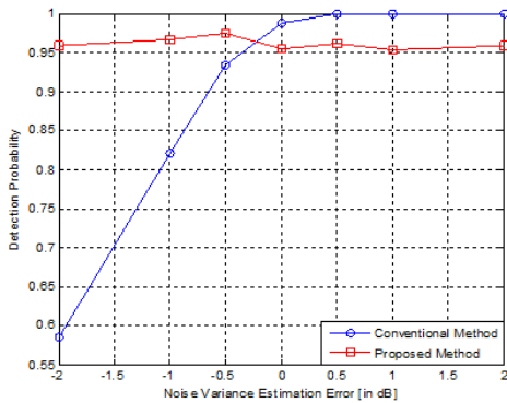
그림 11. 기존 알고리즘과 제안 알고리즘의 검출 성능 모의 실험 결과 Fig. 11. Performance comparison of detection probabilities between the conventional signal detection algorithm and the proposed signal detection algorithm
