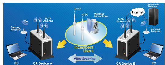
그림 1. TVWS 무선환경 인지 기술 블록도 Fig. 1. Block diagram of cognitive radio technology in TV white space (TVWS)
