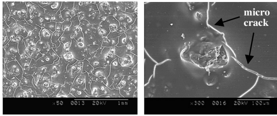
그림 1. 유/무기 복합 세라믹 후처리 적용된 Al-3Mg 용사코팅 층의 표면 형상 Fig. 1. Surface morphologies of Al-3Mg thermal spray coating with sealing treatment of organic & inorganic composite ceramic
