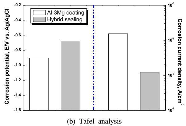
그림 6. 유기/무기 복합 세라믹 후처리 적용dp 따른 Al-3Mg 용사코팅 층의 해수 내 타펠분석 결과 Fig. 6. Results of Tafel analysis in sea water of Al-3Mg thermal spray coating with sealing treatment of organic & inorganic composite ceramic
