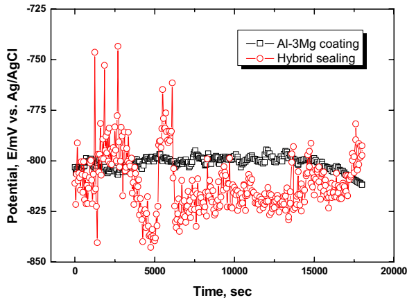
그림 2. 유/무기 복합 세라믹 후처리 적용에 따른 Al-3Mg 용사코팅 층의 해수 내 자연전위 측정 Fig. 2. Potential measurement in sea water of Al-3Mg thermal spray coating with sealing treatment of organic & inorganic composite ceramic
