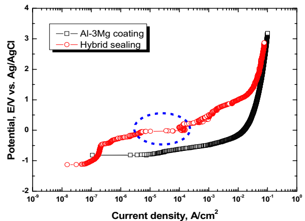
그림 3. 유/무기 복합 세라믹 후처리 적용에 따른 Al-3Mg 용사코팅 층의 해수 내 양극분극 곡선 Fig. 3. Anodic polarization curve in sea water of Al-3Mg thermal spray coating with sealing treatment of organic & inorganic composite ceramic
