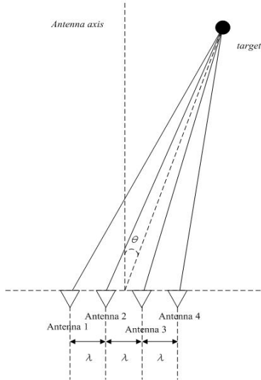
그림 3(a). 선형 배열 위상 비교 모노펄스 안테나 Fig. 3(a). phase comparison monopulse antenna for uniform linear array
