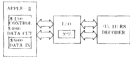
그림 7 실험 구성도 Experimental modeling.
