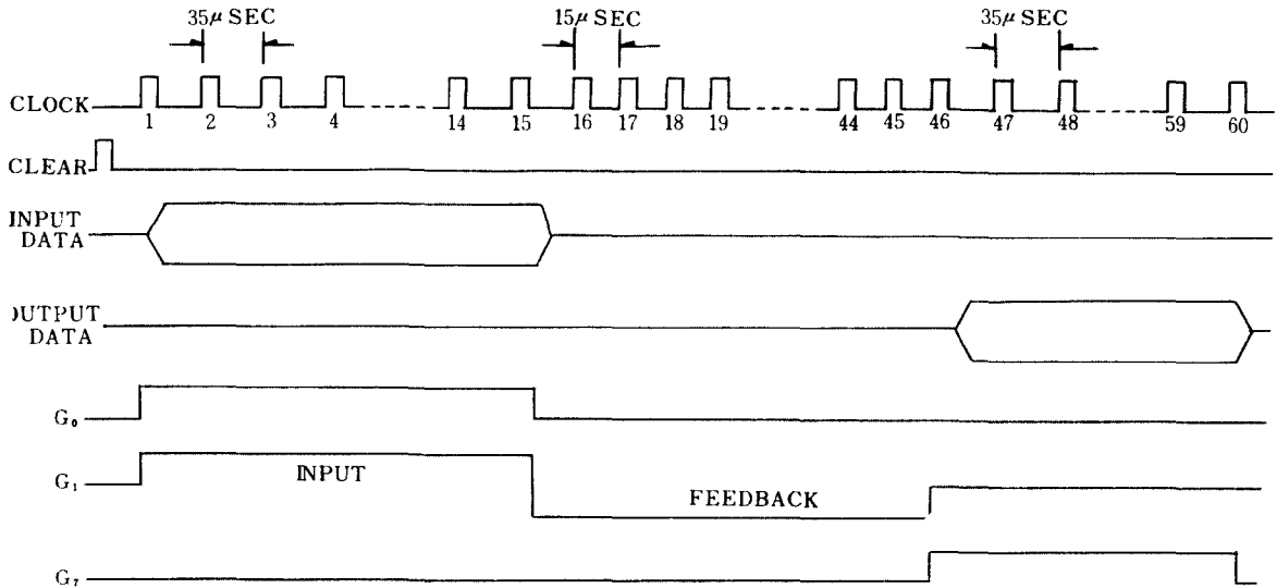
그림 8 디코더 회로의 타이밍 그래프 Timing graph of the decoder circuit.
