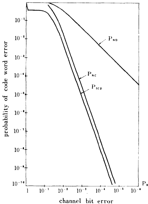
그림 6 (15, 11) RS 코드의 performance 그래프. performance graph of the (15, 11) RS code.
