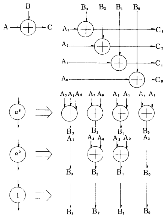
그림 5 Galois Field의 곱셈과 덧셈 예 The example of the Galois Field multiplication and addition.
