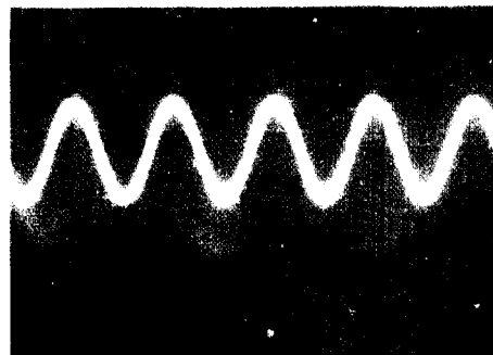
사진 5 발진 주파수 파형 Waveform of SAW osc.
