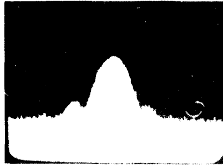
사진 3 SAW소자 주파수 스펙트럼 SAW freq. spectrum.
