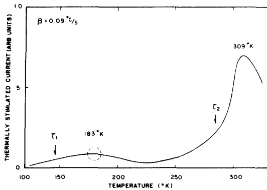
그림 7 溫度上昇 0.09°C/s와 T.S.C. 曲線 Typical conductivity glow curves (T.S.C.) at heating rate of 0.09°C/s.
