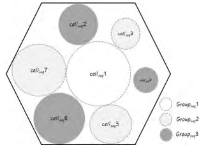
그림 3. 그래프 컬러링 문제 알고리즘을 이용한 영역 그룹화 Fig. 3. Grouping area using graph coloring problem algorithm
