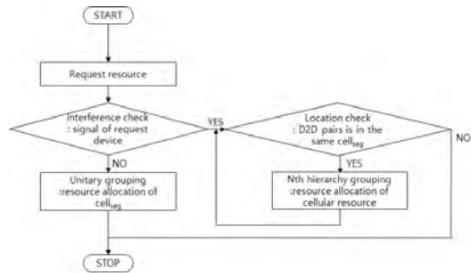
그림 7. 그룹핑 자원 할당 알고리즘 Fig. 7. Grouping resource allocation algorithm
