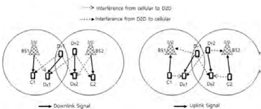
그림 1. 셀룰러 링크와 D2D 링크 간의 간섭 시나리오(좌, 하향링크 자원 재사용, 우, 상향링크 자원 재사용) Fig. 1. Interference scenario between cellular and D2D links(Left, Downlink RB reuse, Right, Uplink RB reuse)
