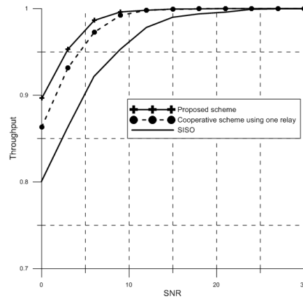
그림 5. 제안된 기법의 throughput Fig. 5. Throughput of the proposed scheme
