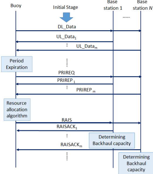
그림 4. 자원분배 프로토콜의 정규 과정 (고정주기 방식) Fig. 4. Normal Stage of resource allocation protocol with fixed period
