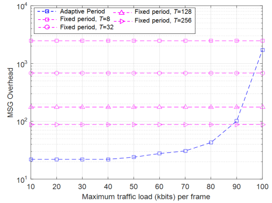
그림 7. 고정주기 및 적응주기 방식의 메시지 오버헤드 Fig. 7. Message overhead of resource allocation protocol with fixed/adaptive period
