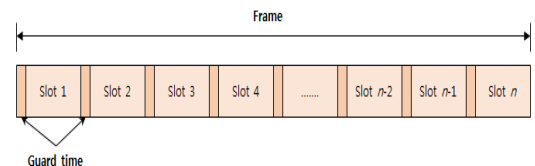
그림 2. TDMA 프레임 구조 Fig. 2. TDMA frame structure
