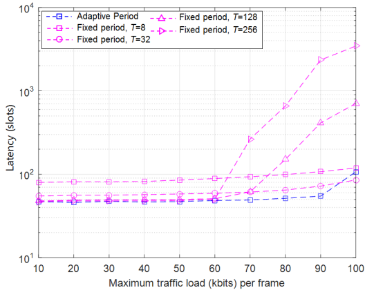
그림 8. 고정주기 및 적응주기 방식의 전송지연 Fig. 8. Queuing delay of resource allocation protocol with fixed/adaptive period
