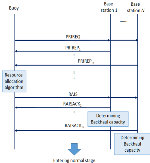
그림 3. 자원분배 프로토콜의 초기 과정 Fig. 3. Initial Stage of resource allocation protocol
