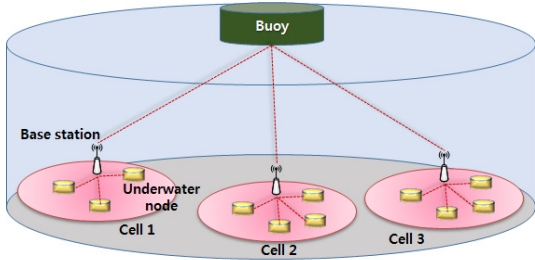
그림 1. 수중 셀룰러 통신 네트워크 구조 Fig. 1. An architecture of underwater cellular communication networks
