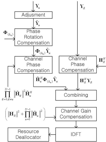
그림 4. 제한하는 상호협력 수신 다이버시티 결합 기법의 블록도
