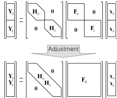
그림 2. MS에서 수신된 신호의 Adjustment 과정 예
